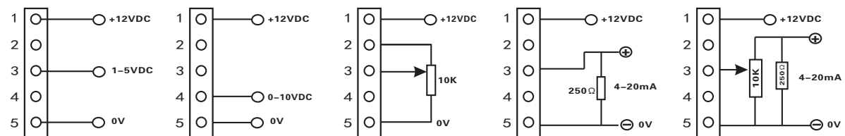
①.1-5V ②.0-10V ③.10K电位器 ④.4-20ma ⑤.限幅4-20ma
