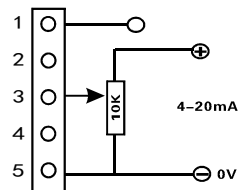
⑤.限幅4-20ma
